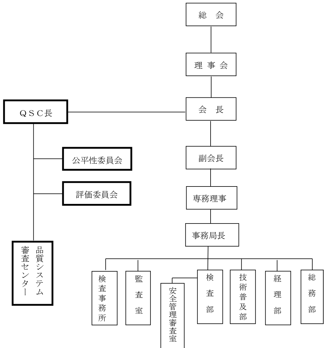
図1 JBAの組織
